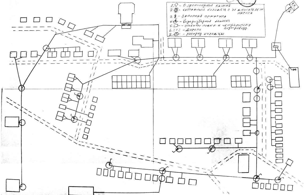
СХЕМА ВОДОСНАБЖЕНИЯ и ВОДООТВЕДЕНИЯ с. СУРУЛОВО
