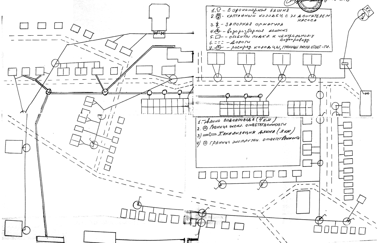
СХЕМА ВОДОСНАБЖЕНИЯ и ВОДООТВЕДЕНИЯ с. СУРУЛОВО
